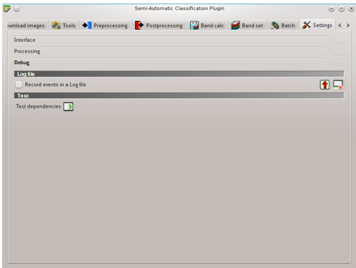
Fig. 23.1: Debug
