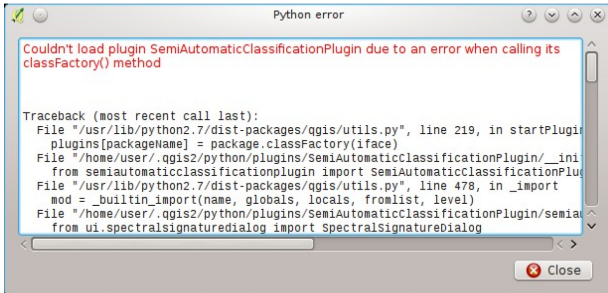
Fig. 23.2: Error message
