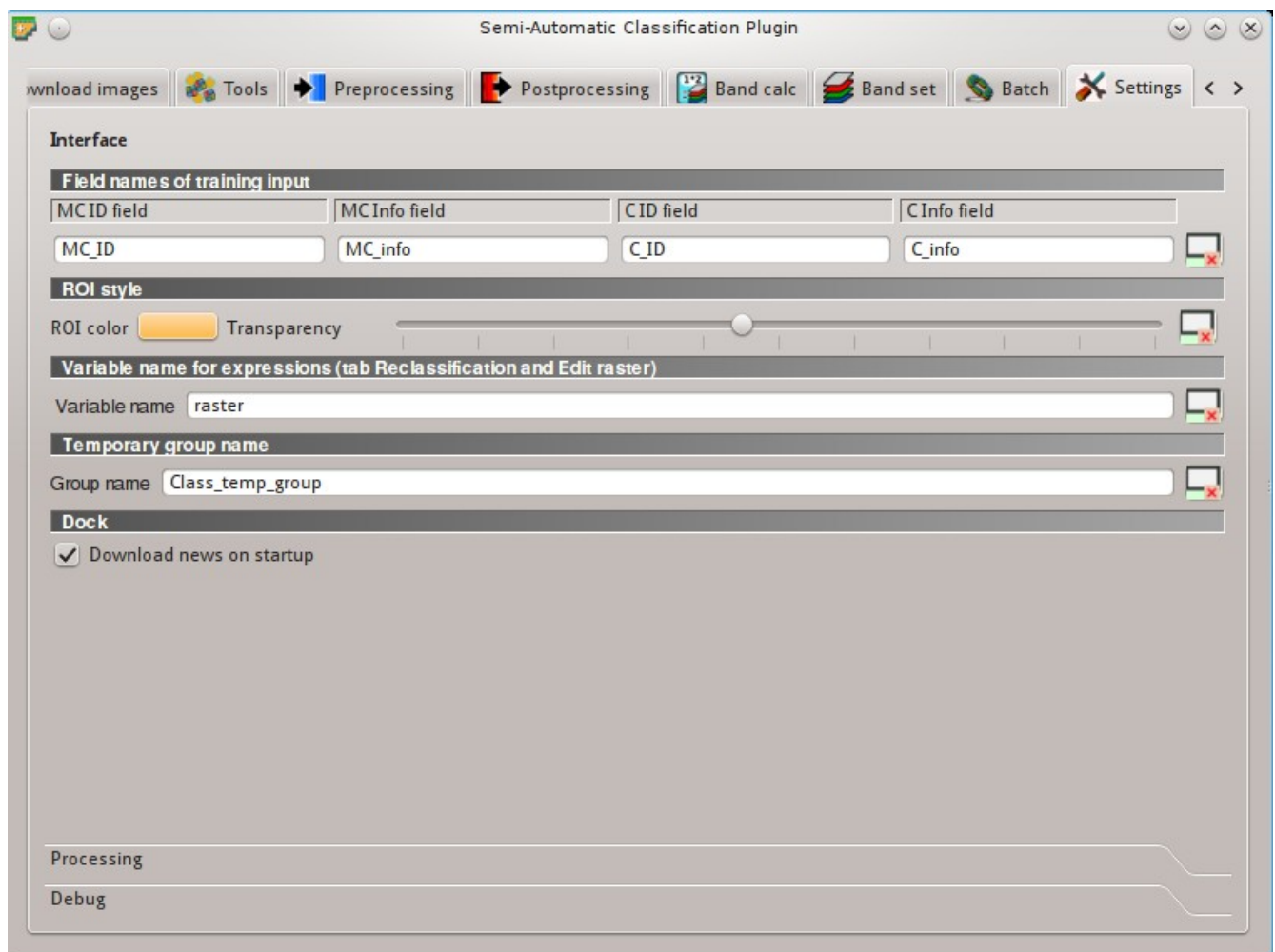
Fig. 10.34: Interface
